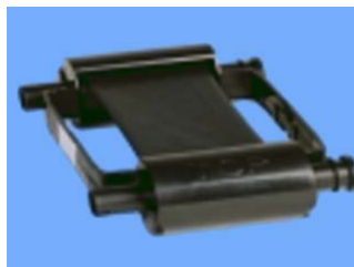
Zebra Monochrom Farbbandkassette (Schwarz), P210, für bis zu 500 Drucke/Kass. Art.-Nr. 10109 – 1 Stück
