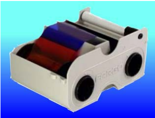
Fargo YMCKO Farbbandkassette, C30, C30 D, DTC, für bis zu 250 Drucke/Kass. Art.-Nr. 14100 – 1 Stück
